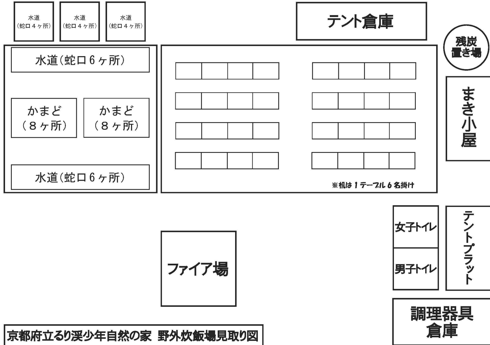
【野外炊飯場平面図】
